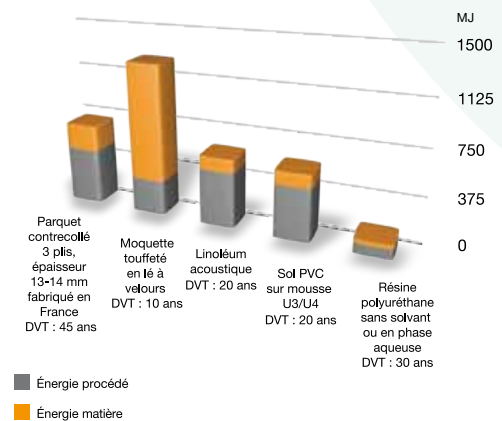
Figure 9 - Comparisons entre énergies primaire totale, énergie procédé et énergie matière pour des revêtements de sol - AILTER, 2011
