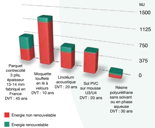
Figure 8 - Comparisons entre énergies primaire totale, énergie renouvelable et non renouvelable pour des revêtements de sol - AILTER, 2011
